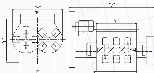
MISTURADORA 120 t/h - 02 CARREGAMENTOS BIG-BAG 1000 kg E 01 SACARIA 50 kg
